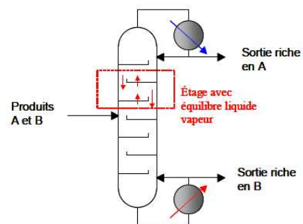
Fig. 2: colonne de distillation
