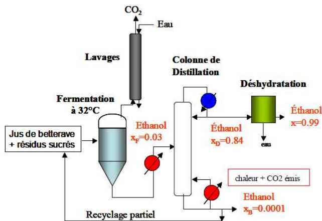
Fig. 1: Schéma de procédé. Fabrication du bioéthanol
